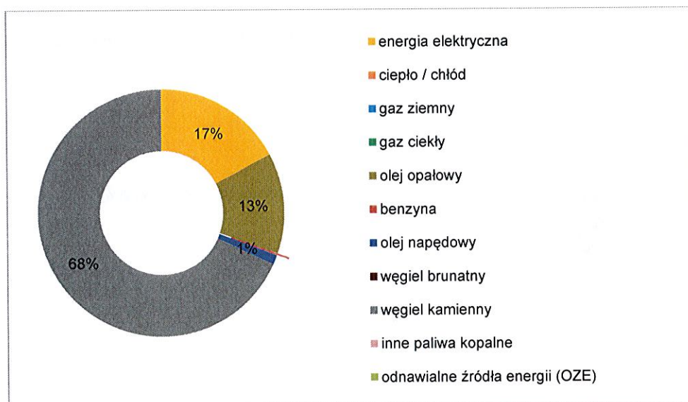
Wykres nr 2: Struktura udziału poszczególnych nośników energii w finalnym zużyciu energii sektora publicznego w roku bazowym [%]
